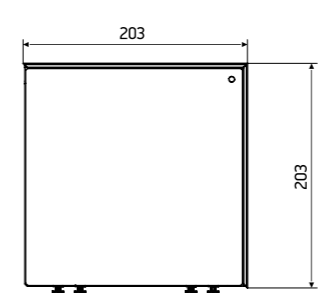
KVU 250-65-90
