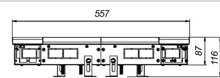
KVU 250-85-135
