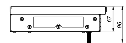
KVU 250-65-90
