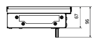
KVU 200-65-90
