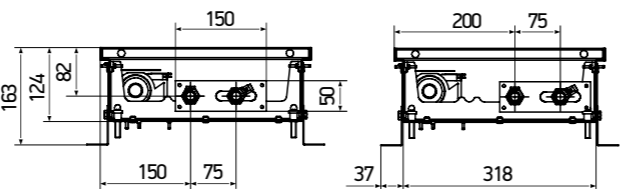
KVZV (KVPV) 350-120
