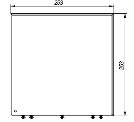
KVU 250-105-90
