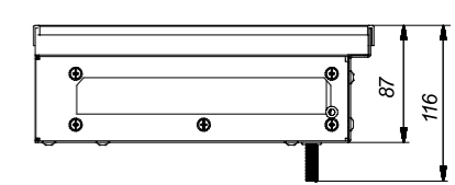
KVU 250-85-90
