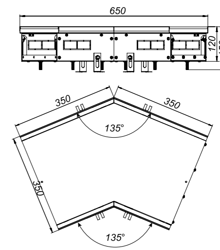
KVU 350-120-135
