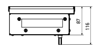
KVU 200-85-90
