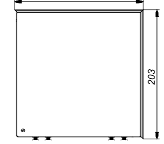
KVU 250-85-135
