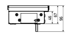
KVU 150-65-90
